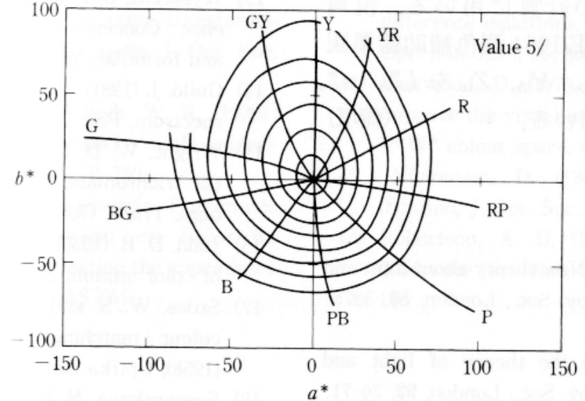
図 4.27 マンセル・バリュ-5 の色票の a^* 値および b^* 値の CIE 1976 a^*b^* 座標面上への置点。(Robertson 46) , 1977)
