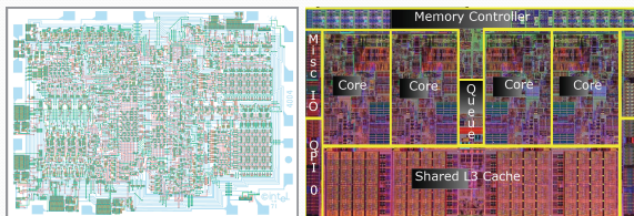
Intel 4004, 1971年 2300トランジスタ 動作クロック: 731kHz
